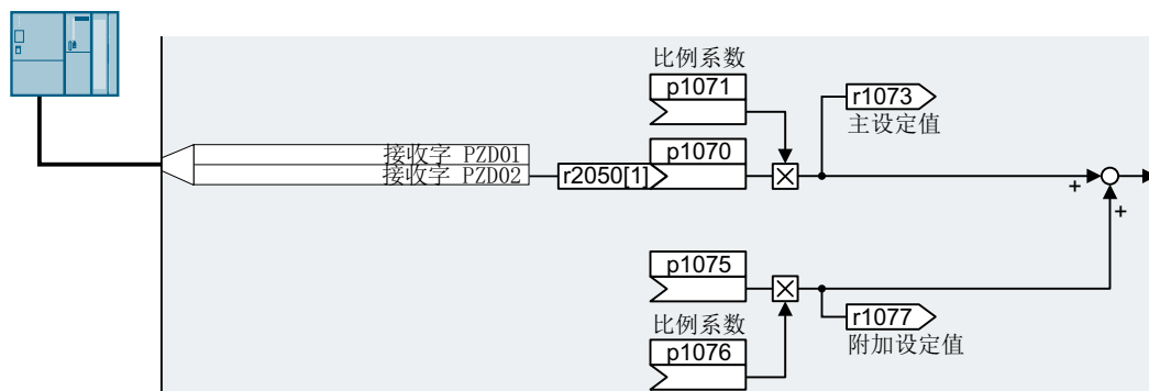
图 6-35 现场总线设为设定值源
