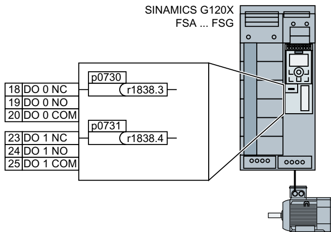
图 6-24 通过数字量输出的反馈信息“STO 生效”
