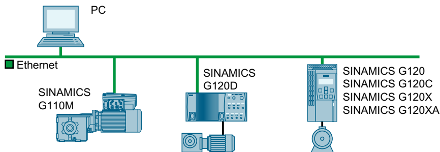
图 4-35 变频器作为以太网节点
