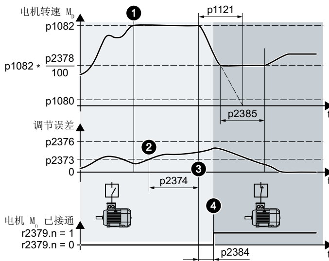
图 6-55 激活非调速电机 M_1 \dots M_2
