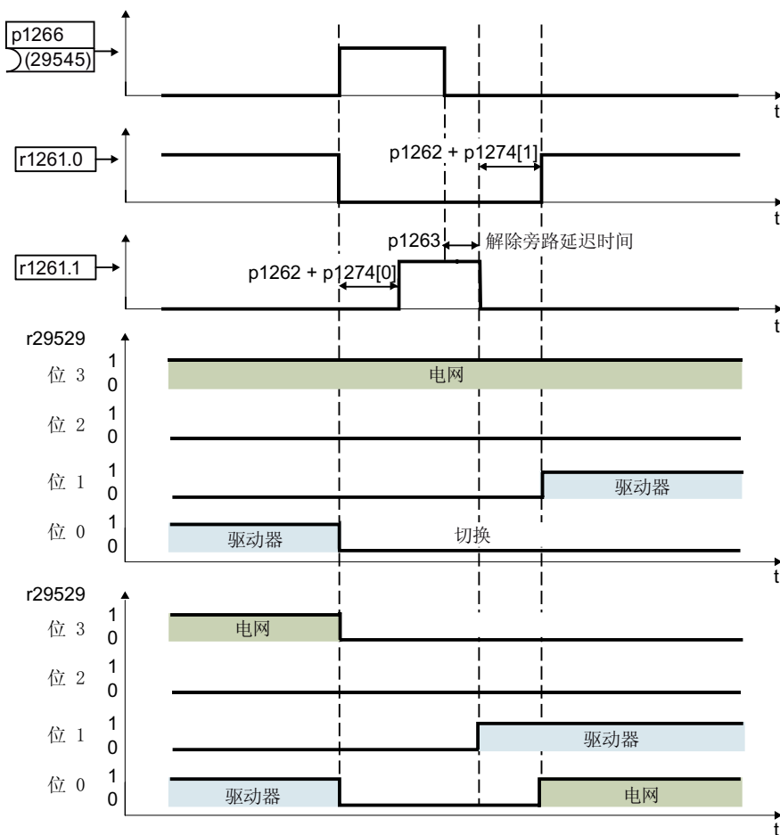
图 6-31 多泵轮换
