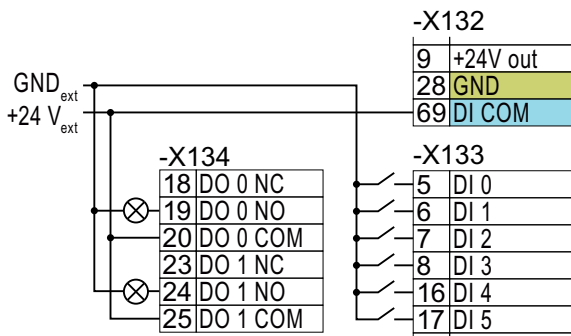
图 4-14 将漏型触点连接到外部电源
