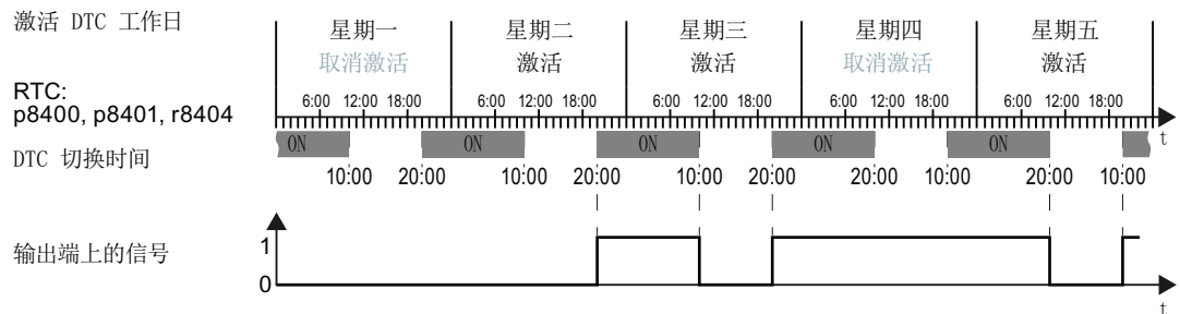
图 6-57 数字时钟的特性示例
