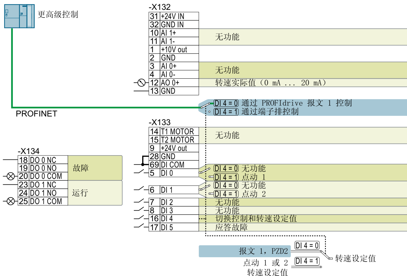
图 4-15 接口的出厂设置
