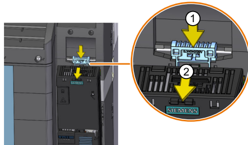
图 4-24 用于“STO”安全功能的端子和开关, 外形尺寸 FSD ... FSG
