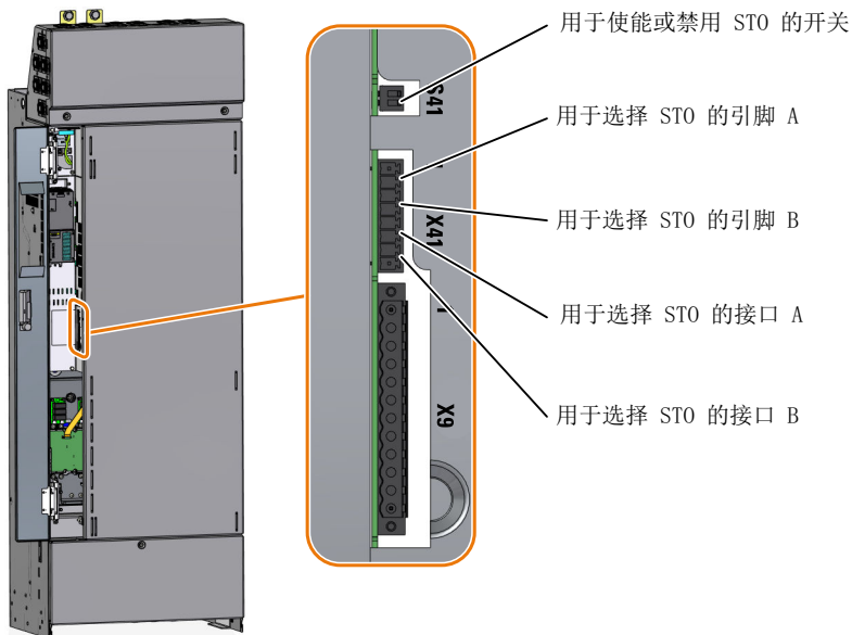
图 4-25 用于“STO”安全功能的端子和开关，外形尺寸 FSH 和 FSJ
