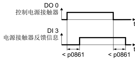
图 6-95 通过 DO 2 的电源接触器控制，带通过 DI 3 的反馈信息
