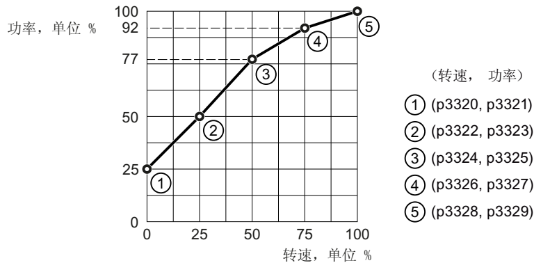
图 6-98 流体特性曲线的出厂设置
