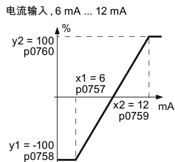
图 6-10 应用示例特性曲线
