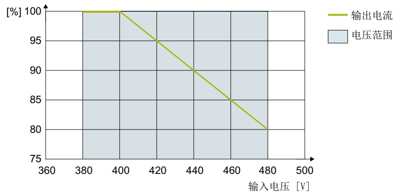
图 11-2 输入电压与电流和电压降容的函数关系，FSH/FSJ
