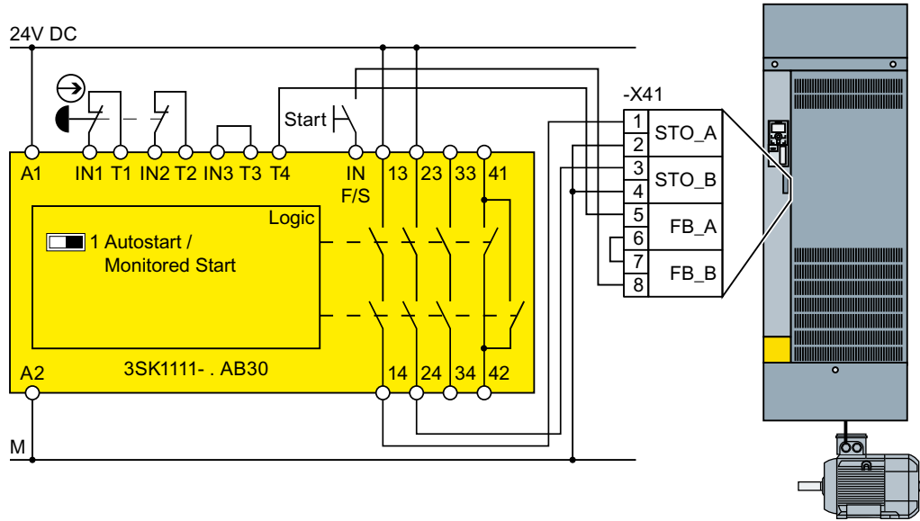
图 4-33 安装在控制柜内的安全继电器的接线
