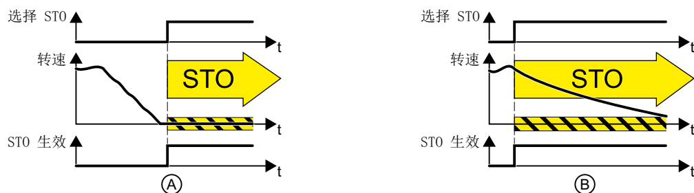
图 6-23 电机在静止 (A) 和旋转 (B) 时的 STO 功能
