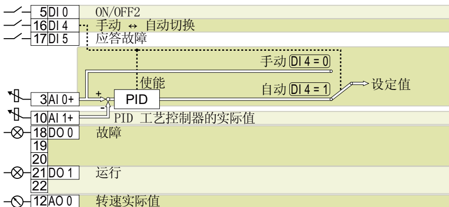
图 4-17 默认设置 42: “PID 模拟量控制”
