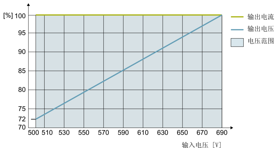
图 11-3 输入电压与电流和电压降容的函数关系，FSA..FSG
