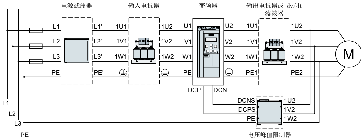
图 4-5 连接变频器 FSH/FSJ 及其选件
