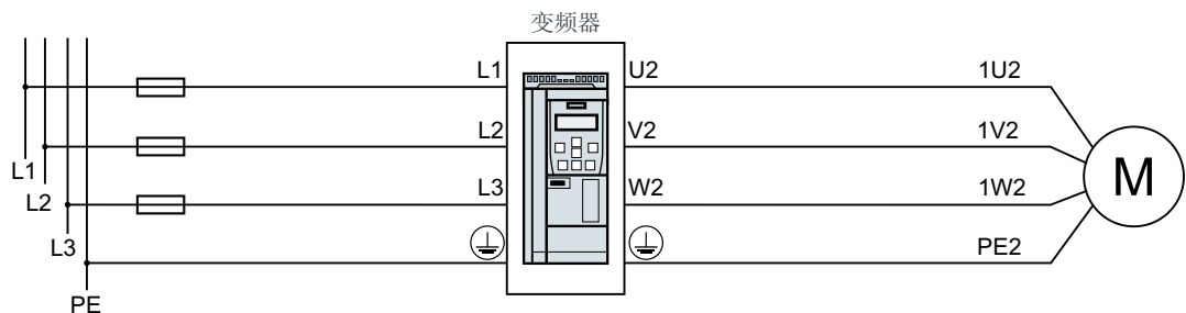
图 4-4 连接变频器 FSA ... FSG 及其选件
