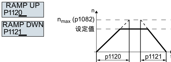
图 5-10 电机的斜坡上升和下降时间
