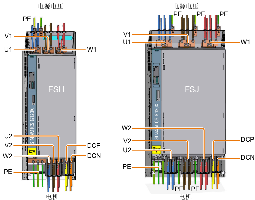
图 4-11 电源端子、电机端子和直流母线端子
