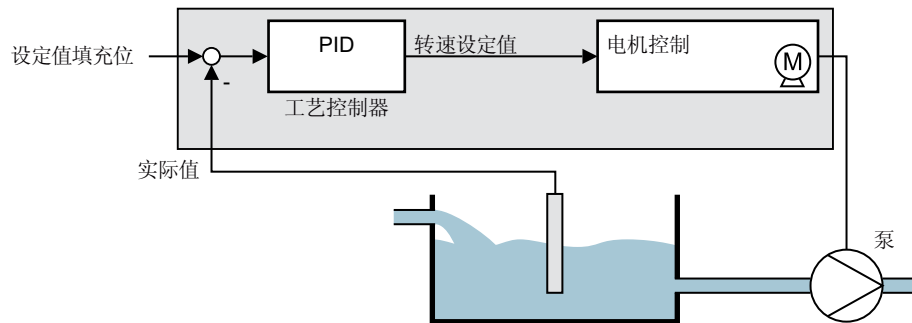
图 6-47 示例：工艺控制器用作流量控制器
