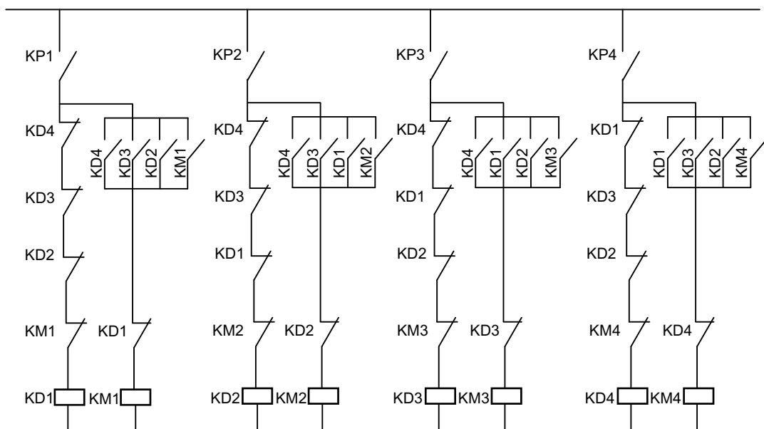
图 6-25 主电路
