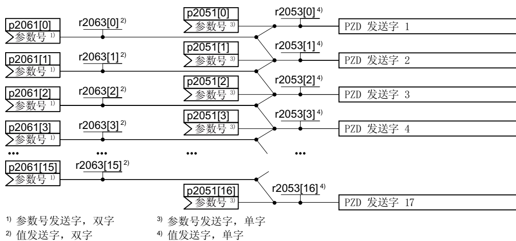
图 6-20 发送数据的互联
