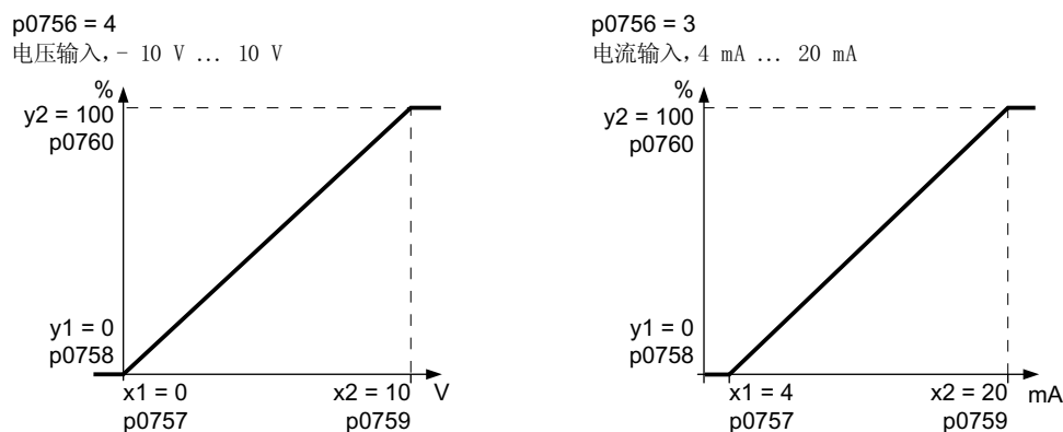
图 6-9 定标特性曲线示例
