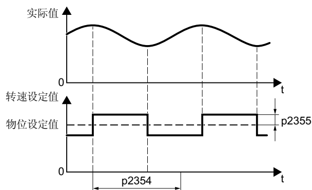
图 6-50 自动优化时的转速设定值和过程实际值示例
