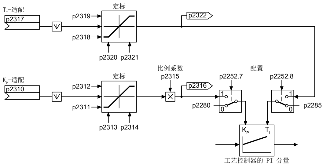
图 6-51 控制器匹配
