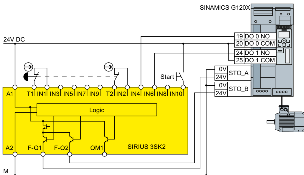
图 4-29 安装在控制柜内的安全继电器的接线
