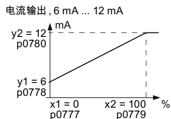
图 6-13 应用示例特性曲线
