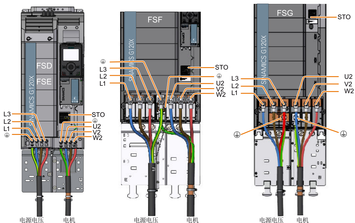
图 4-9 连接电源和电机
