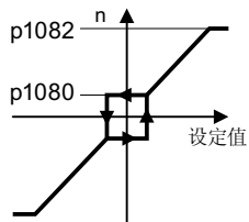
图 5-7 电机的最小转速和最大转速
