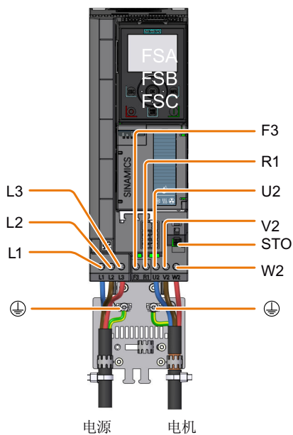
图 4-6 连接电源、电机和直流母线端子
