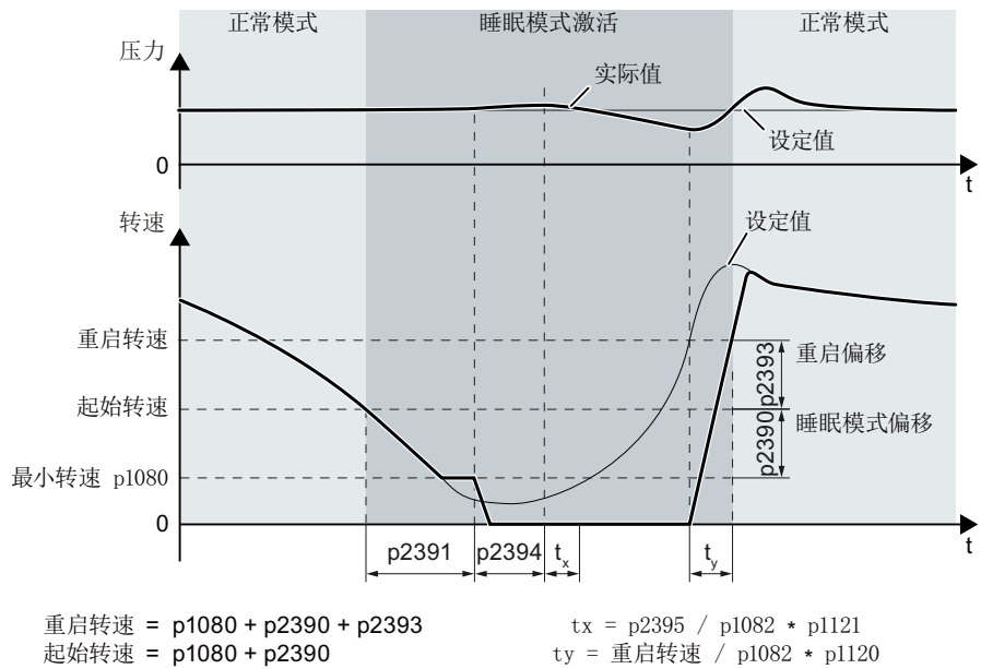
图 6-93 通过外部设定值且不带升速的睡眠模式
