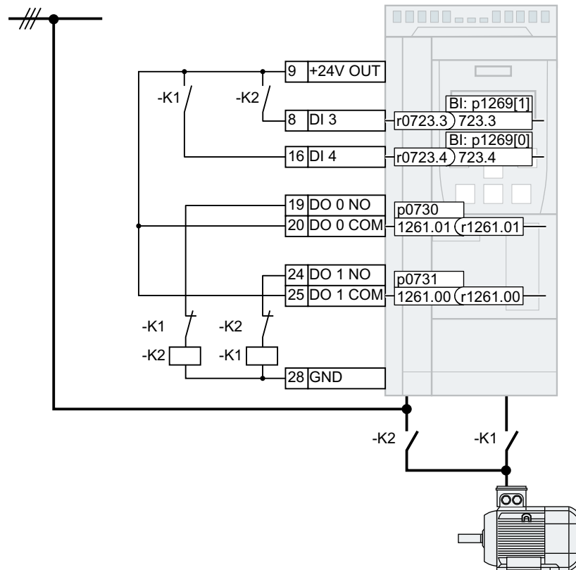
图 6-87 由变频器进行的旁路控制
