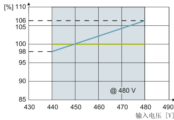
图 11-1 输入电压与电流和电压降容的函数关系，FSA ... FSG
