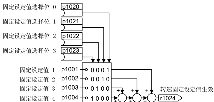
图 6-40 转速固定设定值的直接选择
