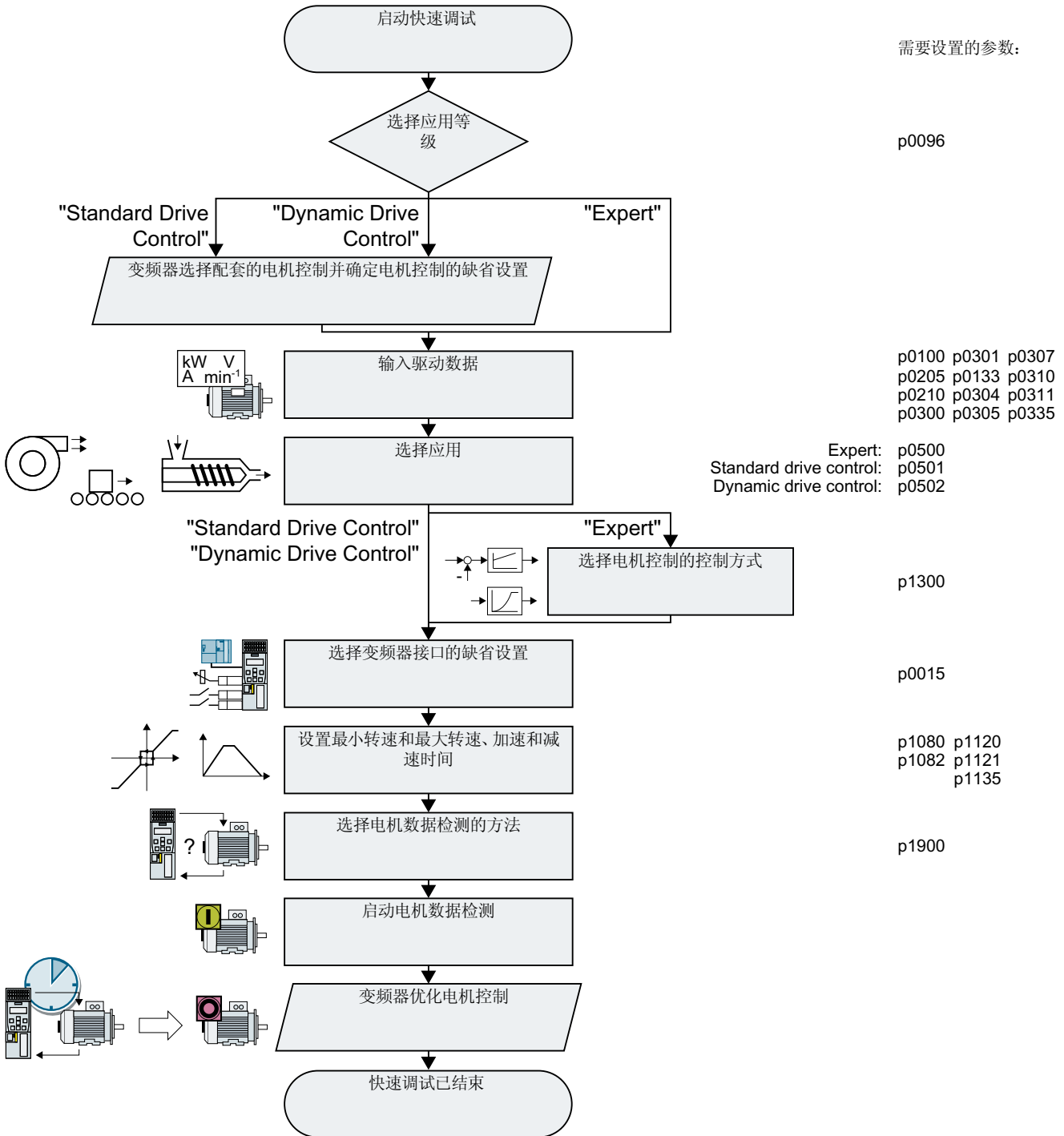
图 5-6 使用操作面板 BOP-2 进行快速调试
