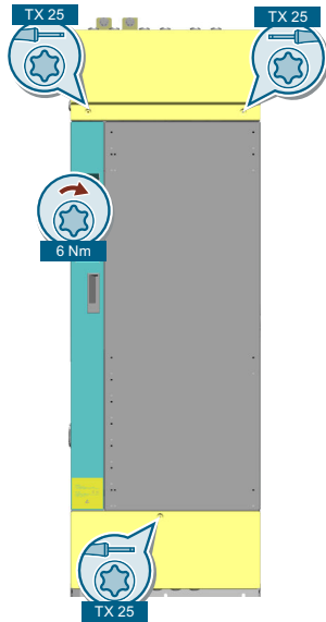
图 4-10 拆下前盖板
