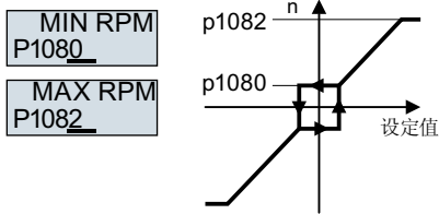
图 5-9 电机的最小转速和最大转速
