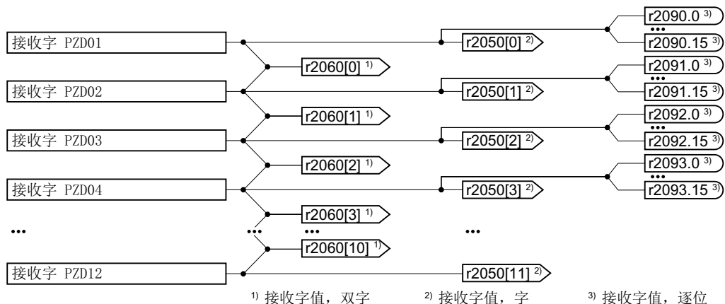
图 6-21 接收数据的互联
