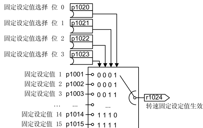
图 6-41 转速固定设定值的二进制选择
