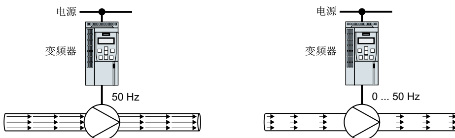
图 6-97 使用泵和变频器的流体控制
