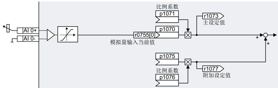
图 6-34 示例：模拟量输入 0 设为设定值源
