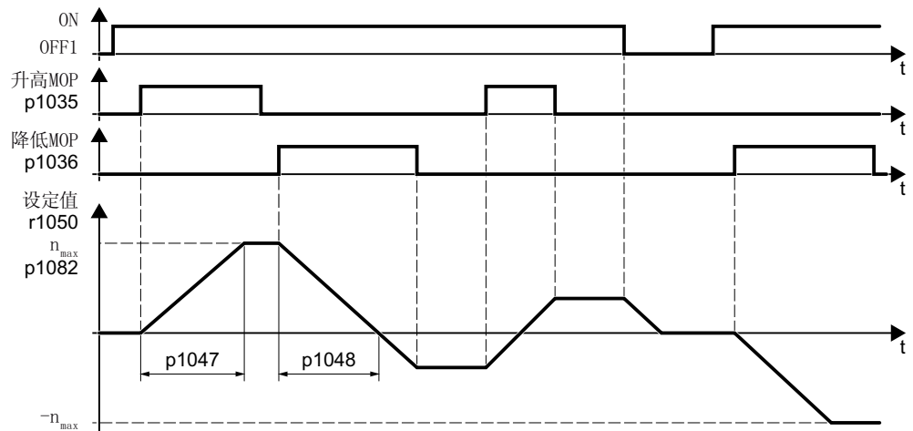
图 6-37 电动电位器的功能图
