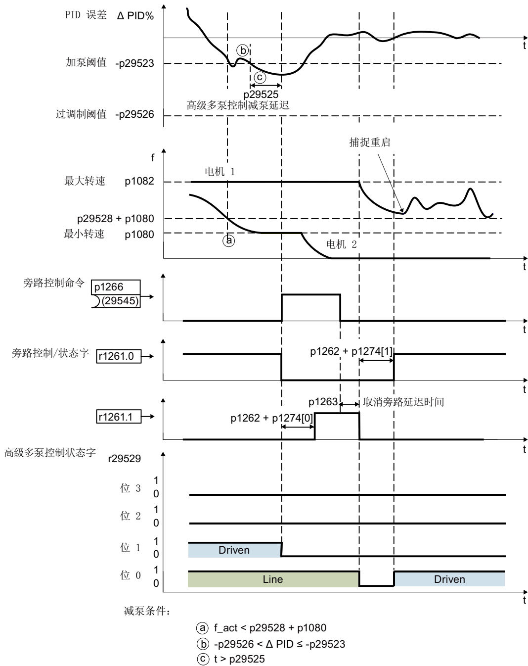
图 6-28 基于固定顺序减泵 ( p29522 = 0 )
