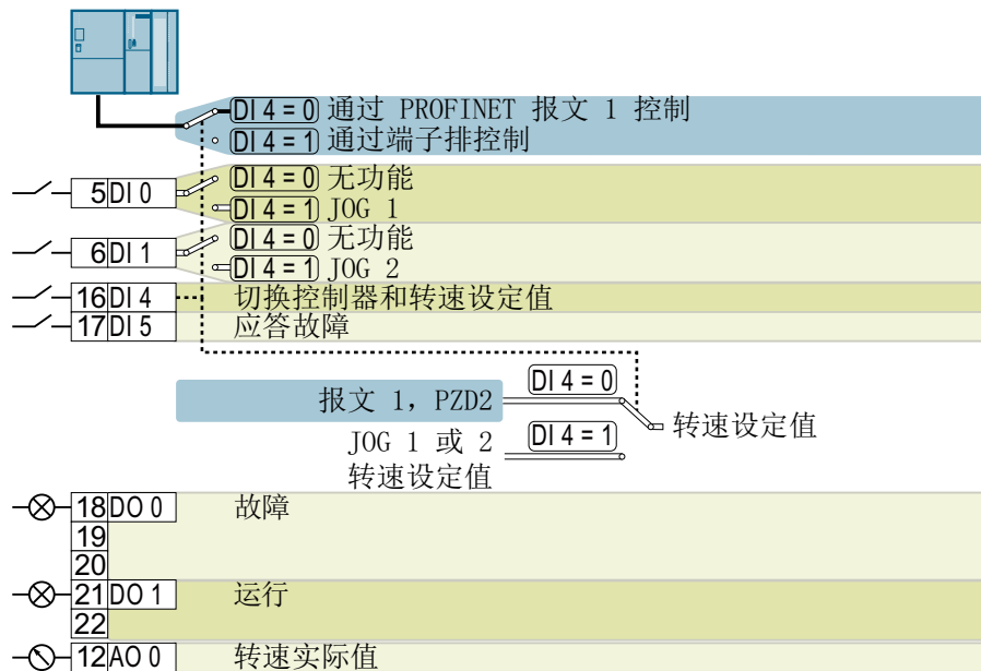
图 4-19 默认设置 57: “PROFINET 控制”
