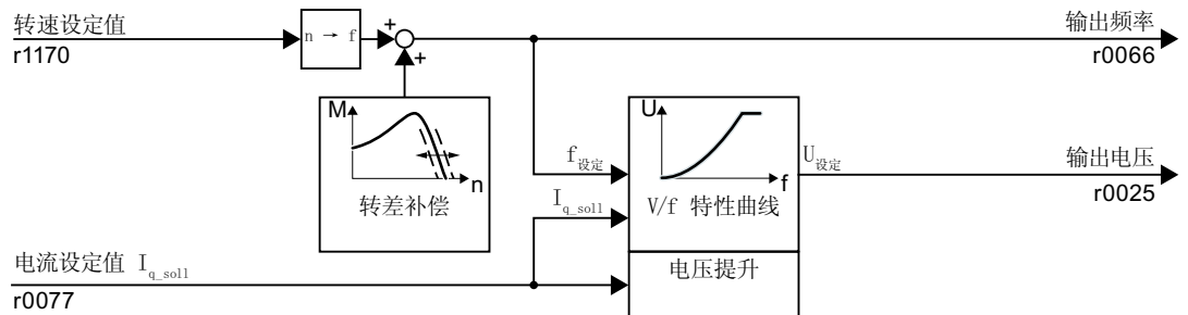
图 6-64 选择 Standard Drive Control 后的 V/f 控制的预设置
