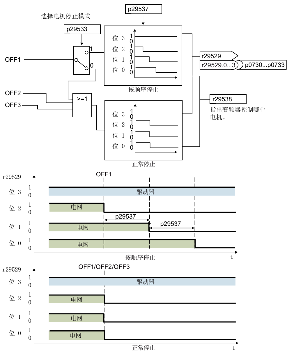
图 6-30 停机模式
