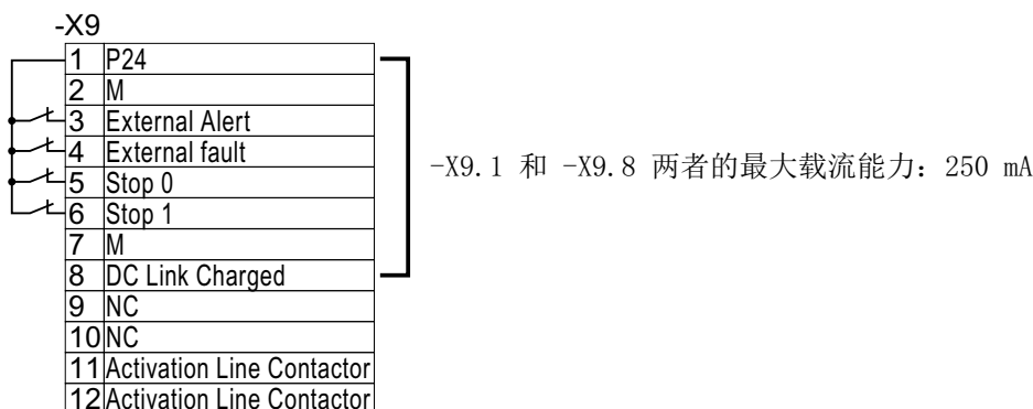
图 4-22 端子排 X9, 提供内部 24 V 电源
