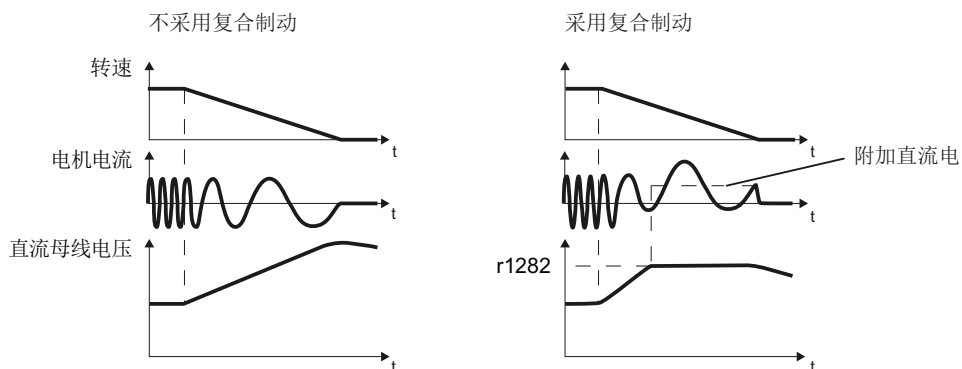
图 6-71 电机制动：无复合制动，有复合制动
