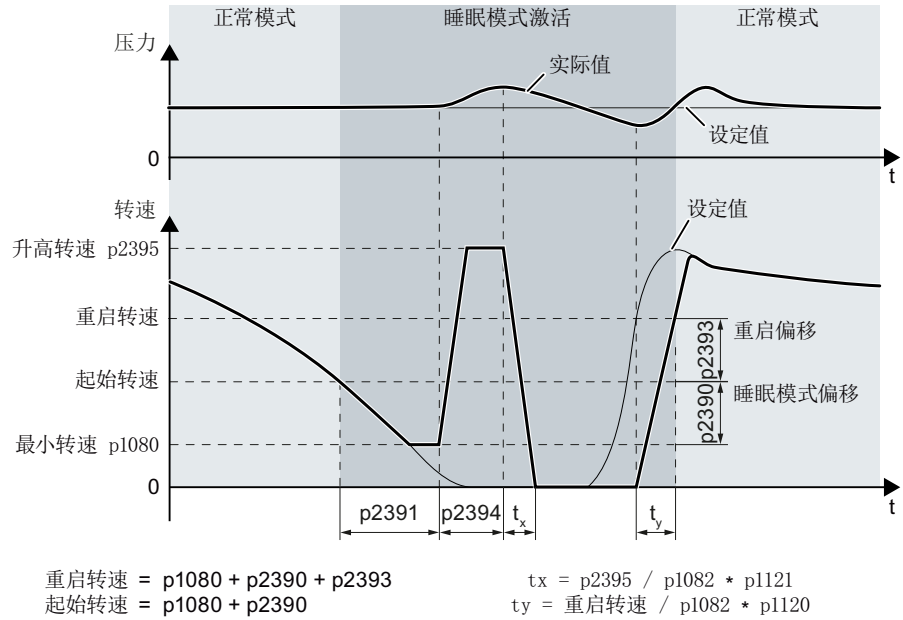
图 6-92 设定值由外部给出且带升速的睡眠模式
