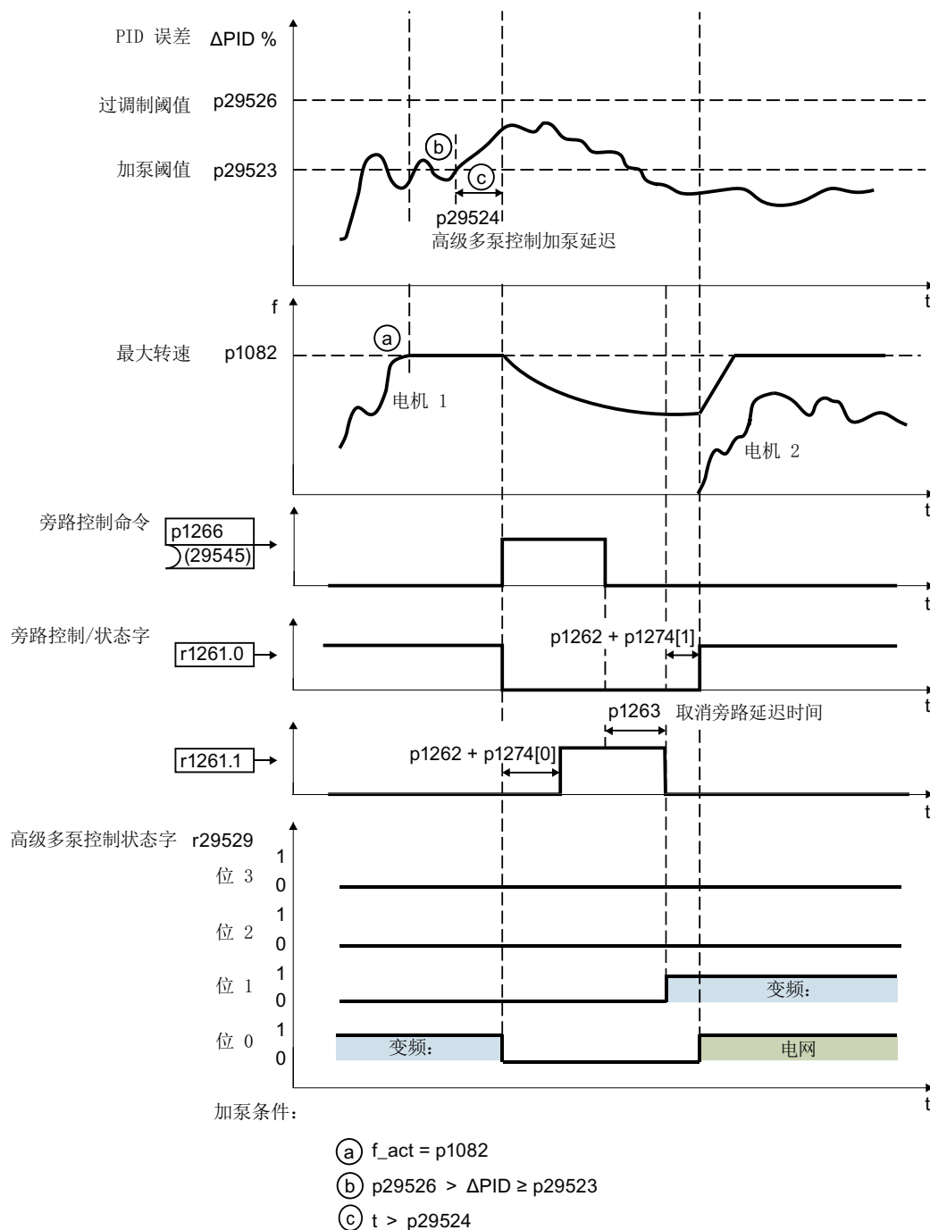
图 6-27 加泵
