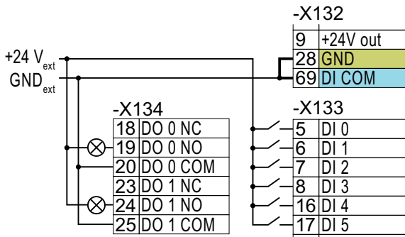
图 4-13 将源型触点连接到外部电源
