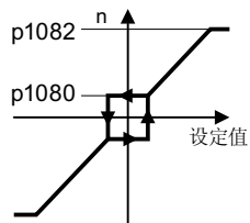
图 5-11 电机的最小转速和最大转速
