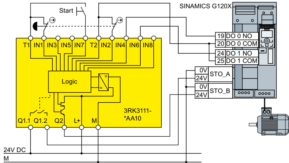
图 4-27 安装在控制柜内的模块化安全系统的接线示例
