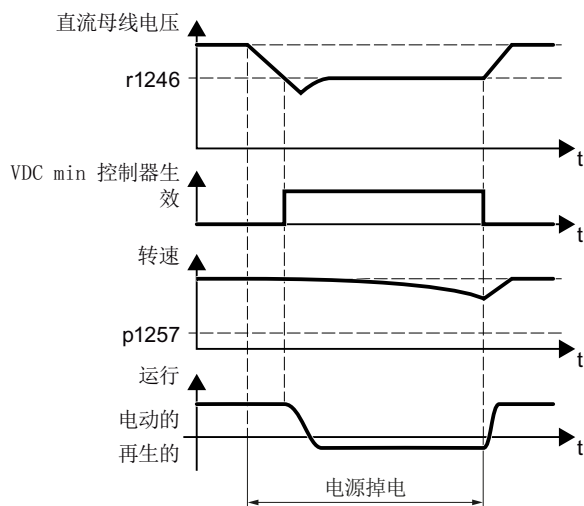
图 6-80 动能缓冲的工作原理
