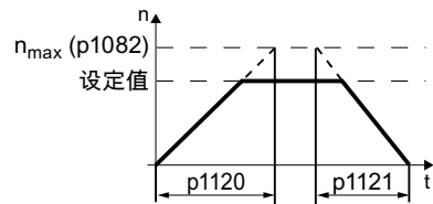
图 5-8 电机的斜坡上升和下降时间
