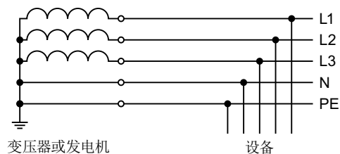
图 4-1 TN 系统
