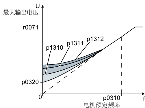
图 6-66 线性特性曲线上的升压降低示例
