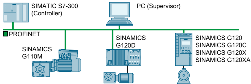
图 4-34 变频器在 PROFINET IO 模式中
