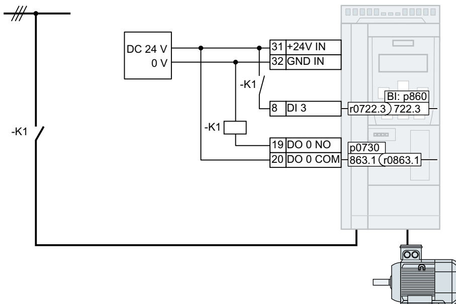
图 6-94 通过 DO 0 的电源接触器控制，带通过 DI 3 的反馈信息
