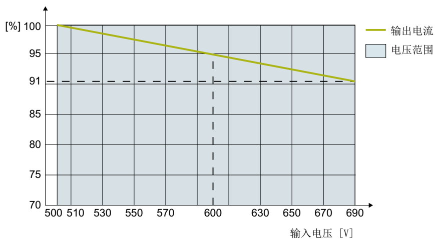
图 11-4 输入电压与电流和电压降容的函数关系，FSH/FSJ
