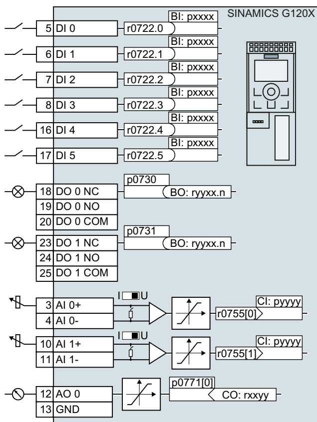
图 6-4 输入和输出的内部互联
