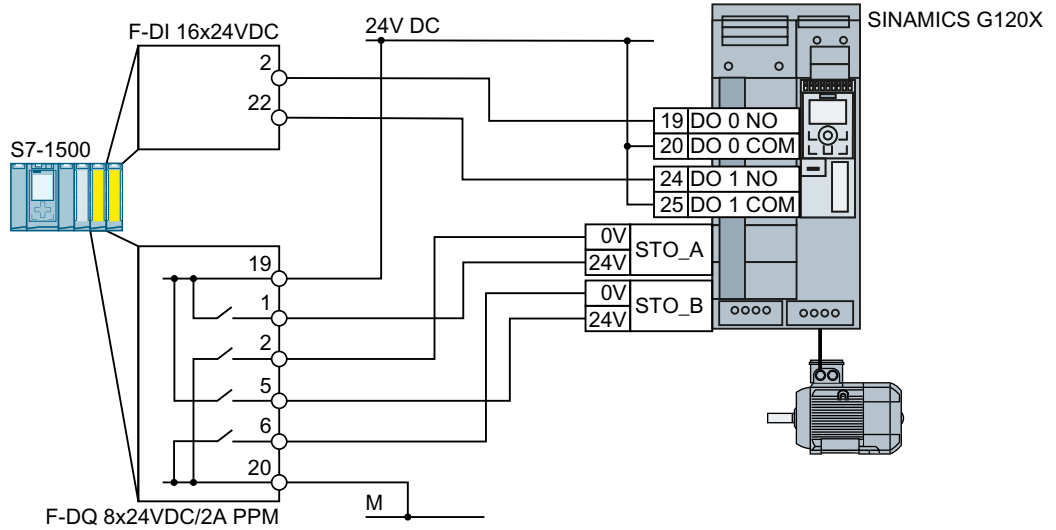
图 4-31 安装在控制柜内的 SIMATIC S7-1500 的接线
