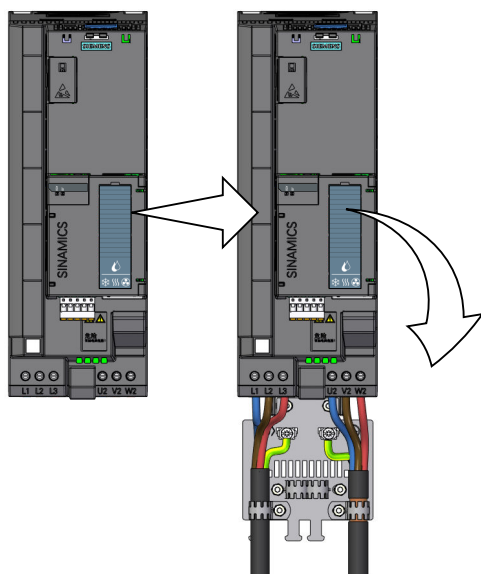
图 10-1 更换受损变频器
