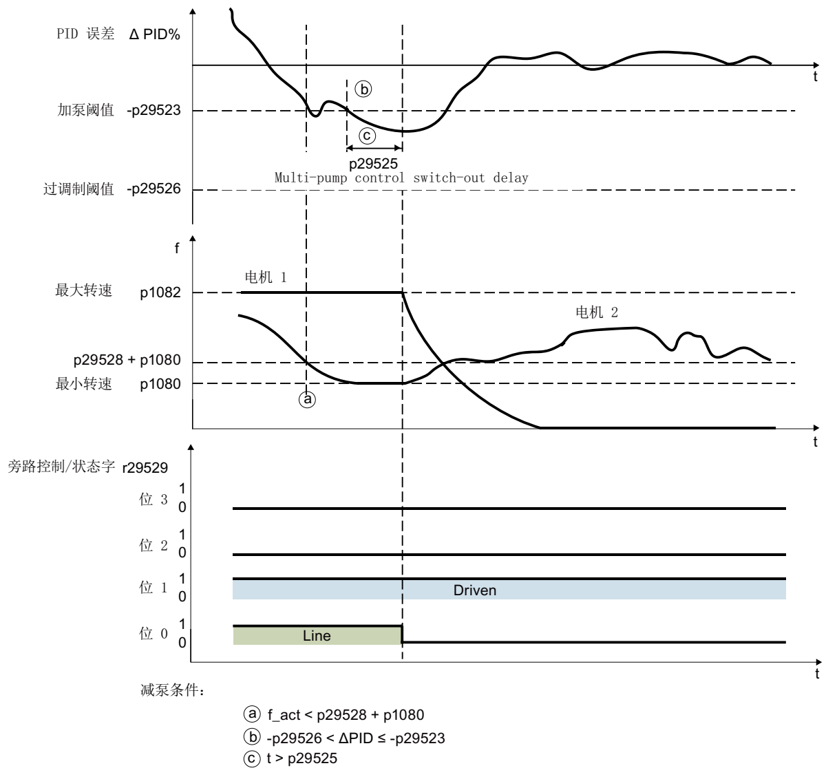
图 6-29 基于绝对运行时间减泵 (p29522 = 1)
