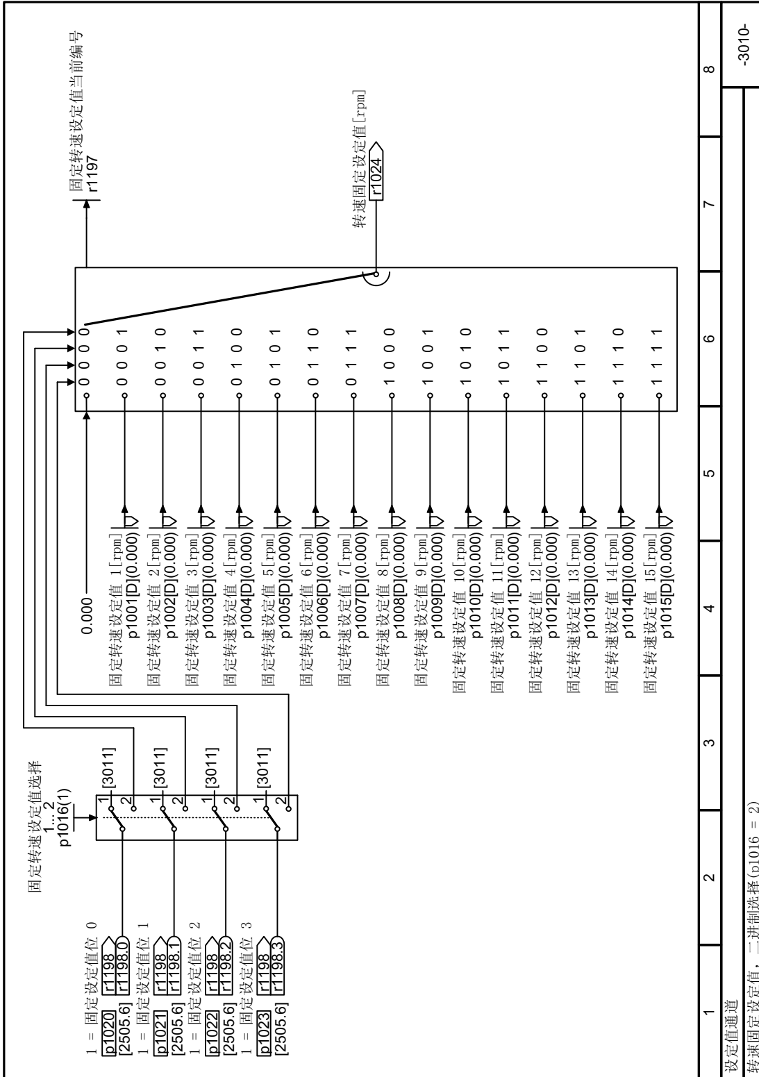
图 6-42 转速固定设定值, 二进制选择
