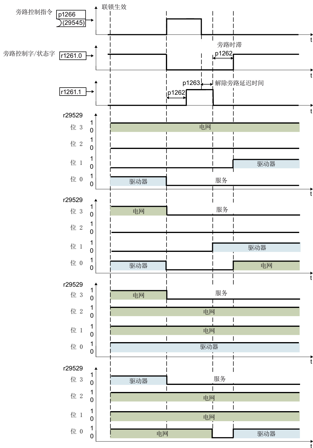
图 6-32 维修模式
